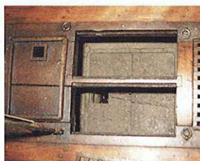
Grandes écoutes. Celle du second pont est à deux volées de caillebotis, avec une entremise centrale amovible. Celle du premier pont est fermée par deux grands panneaux, avec un écouillon pour l'ancre de miséricorde. Sur la gauche, apparaissent l'ouverture pour l'évacuation des fumées du four à pain et le cadre pour l'eau de refroidissement du pont, en cas de besoin.
