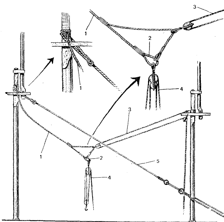
Fig. 414. Paranco di straglio. 1. Penzolo a colonna; 2. gassa del penzolo; 3. ghia; 4. paranco; 5. straglio di maestra.
