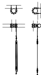
Grote marsera Main topsail yard Großmarsrah
