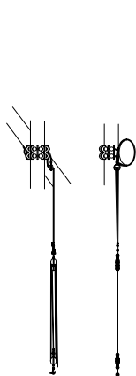
Bezoansroede Mizzen yard Besenrute
